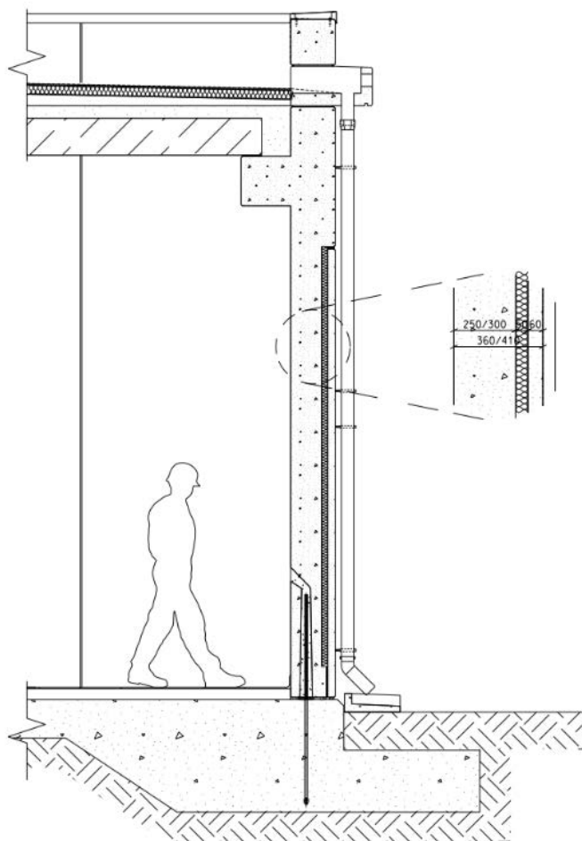
Figura 19. Sección constructiva por panel prefabricado de fachada.
