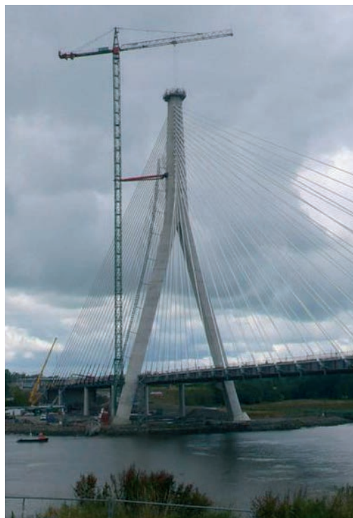
Pilono del Puente de Waterford (Irlanda) en construcción
