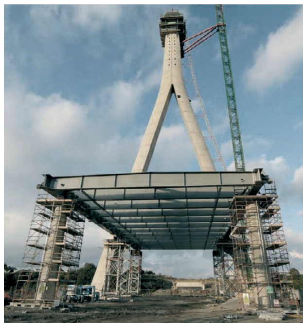
Figura 36. Montaje de estructura metálica en vanos traseros. Figure 36. Installation of steel structure in back spans.
