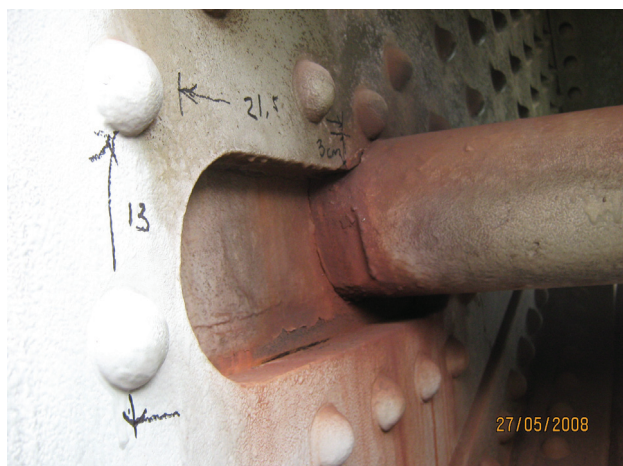
Figura 15. Estado original de los bulones de 5" Figure 15. 5" pins original condition
