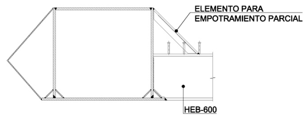
Figura 17. Detalle del empotramiento parcial de las vigas transversales en la viga longitudinal
