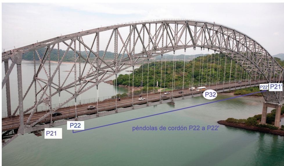
Figura 48. Vista del puente con la numeración de las péndolas extremas y medias Figure 48. View of the bridge with the number of the central and end hangers
