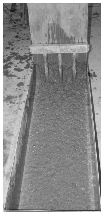
Figura 2. Resultado final del ensayo de la caja en L
