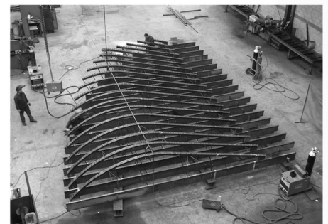
Cubierta del Ayuntamiento de Cabanillas (Madrid)
