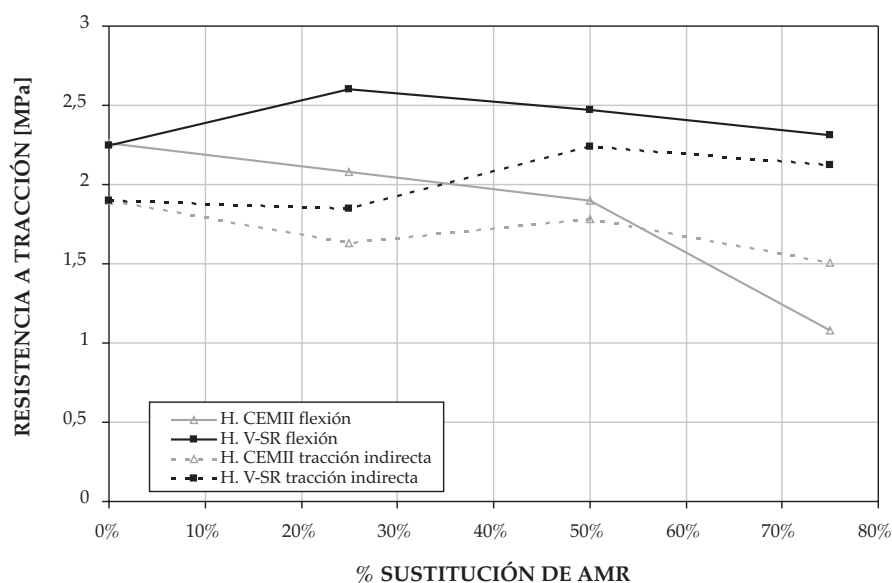
Figura 8. Resistencia a tracción en función del % de AMR.
