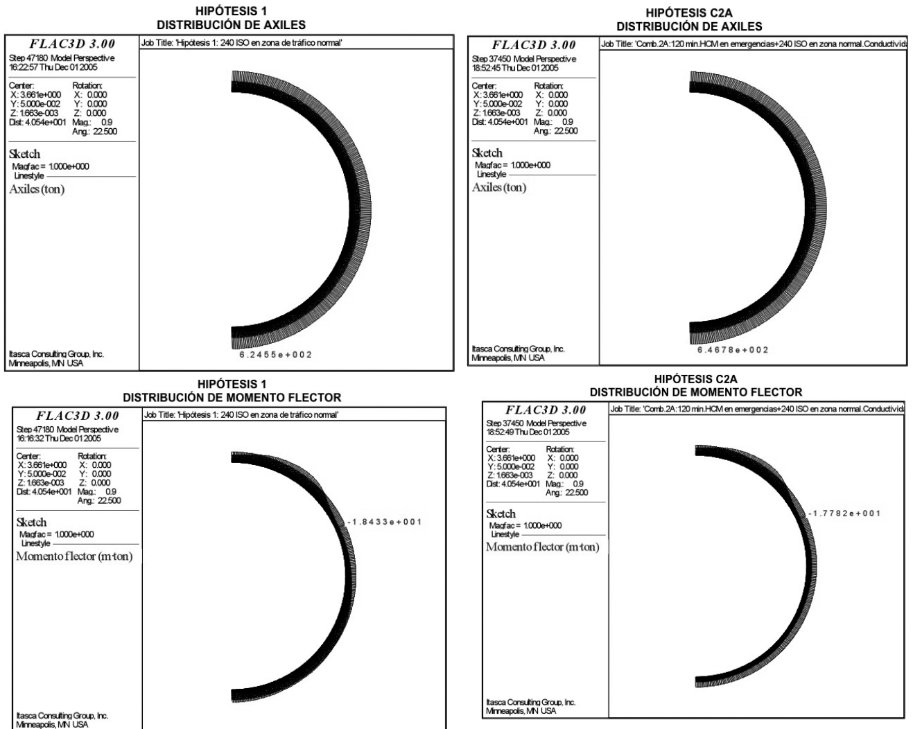
Figura 26. Resultados del análisis mecánico del anillo.
