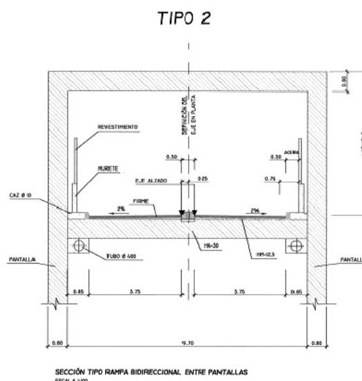
Figura 9. Sección Tipo 2.
