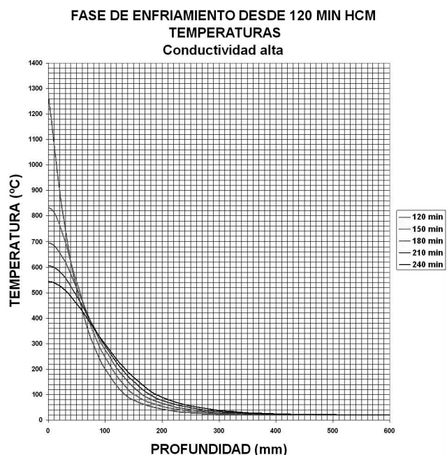
Figura 24. Exposición al fuego de las dovelas del anillo. Enfriamiento. Temperaturas alcanzadas a diferentes profundidades.
