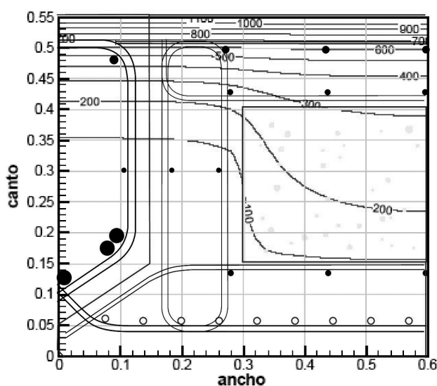
Figura 28. Resultados del análisis térmico de la losa. Isotermas tras 240 minutos de exposición a ISO 834 por cara superior.
