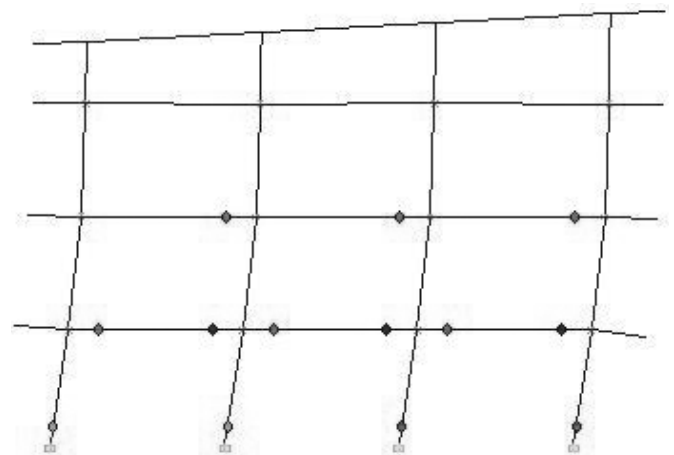
Figura 12. Condición estructural en el umbral del estado de daño severo.
