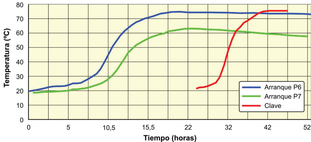
Figura 21. Evolución de las temperaturas del hormigón en arco 2. Figure 21. Variation in concrete temperature in arch 2.
