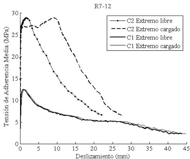
Figura 5. Curvas tensión de adherencia media-deslizamiento para probetas con acero.
