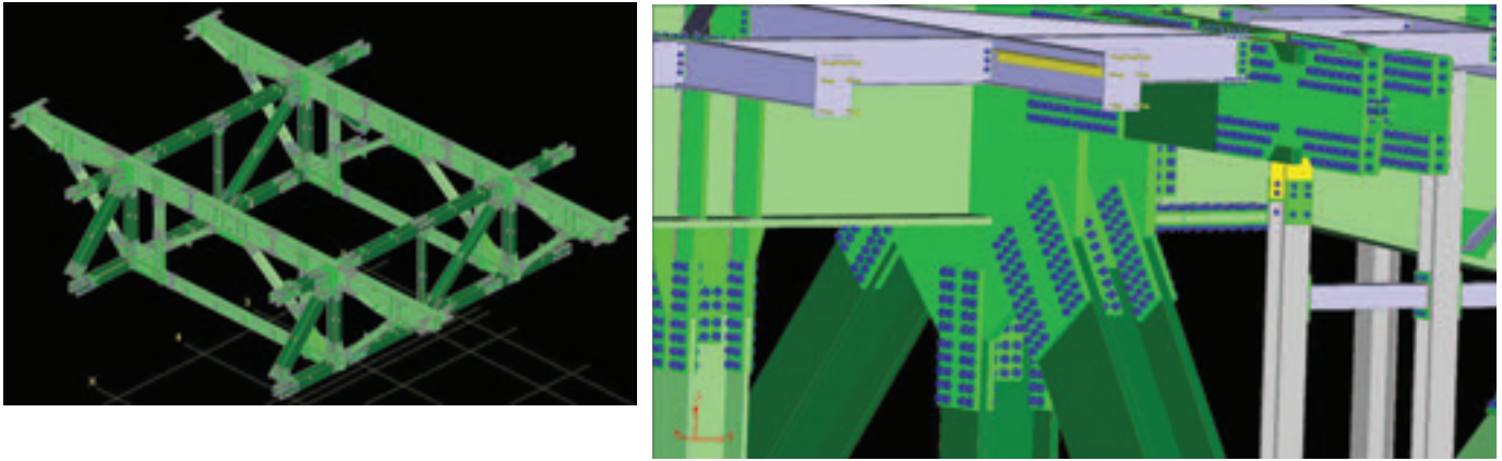
Figura 19. Vistas del modelado 3D de la estructura para el proyecto de taller. Figura 19. Three-dimensional modelling of the structure for shop drawings.
