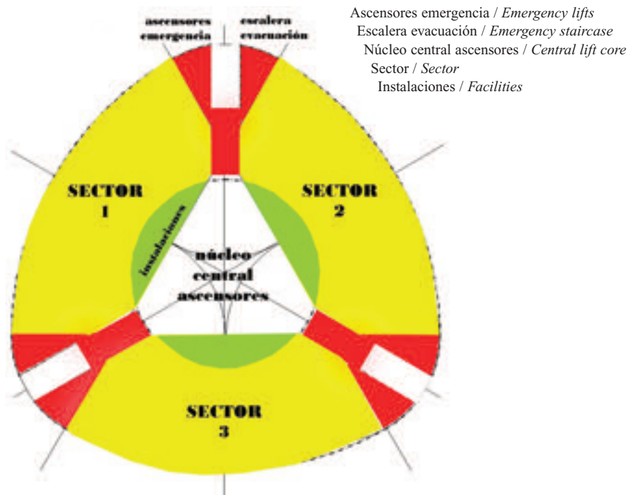
Figura 13. Sectorización frente a incendios y distribución de escaleras de evacuación y ascensores de emergencia.
