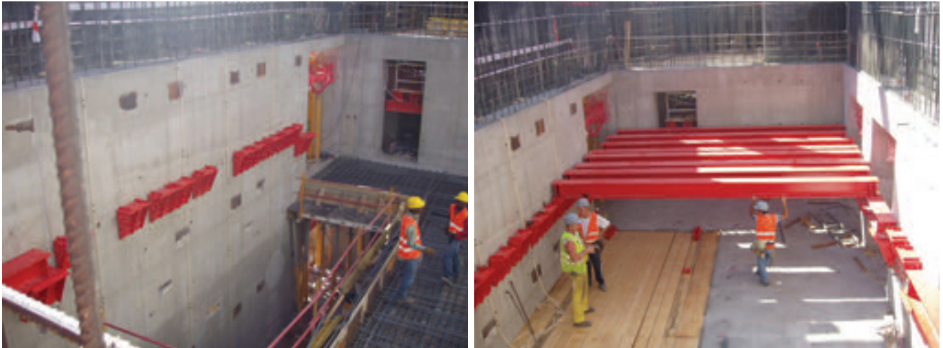
Figura 15. Estructura soporte del encofrado de losa de 1,90 m. Figure 15. Shoring for the 1.90-slab formwork.
