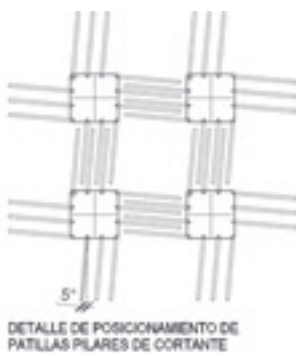
Figura 2. Disposición de armadura de torretas de cortante y plantilla de armadura. Detalle de paso de armadura longitudinal inferior entre las barras verticales de las torretas de cortante, en zona de solapo.
