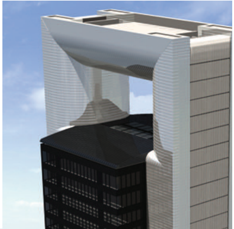
Figura 13. Geometría de la coronación de núcleos Figure 13. Core crown geometry.
