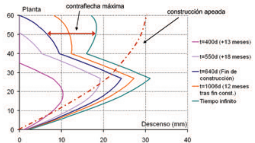
Figura 22. Descensos diferenciales entre el núcleo central y los soportes principales a lo largo de la vida del edificio. Figure 22. Differential drops between the central core and the main supports throughout the building's lifetime.
