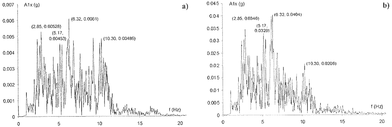
Figura 7. Transformadas de Fourier correspondientes a la aceleración en la parte superior de la estructura, para distintas escalas de la excitación: a) FE = 0.353 , b) FE = 2.238 .
