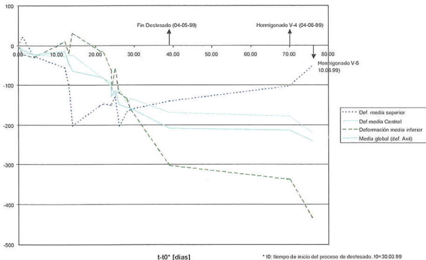
Figura 10. Deformaciones en dovela de cierre debidas al desfasado de los cables y el hormigonado de los vanos 4 y 5. Figure 10. Strains in closing segment due to the loosening of the cable stays and the concreting of the arch deck.
