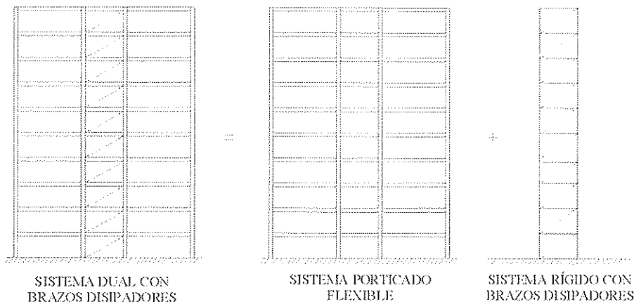
Figura 1. Sistema dual avanzado con disipadores de energía.
