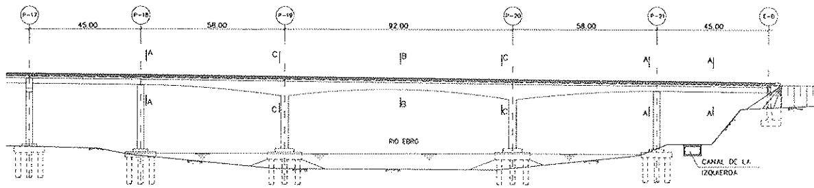
Figura 3. Alzado.
