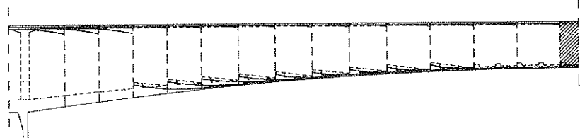
CABLES TIPO "A" (FASE ISOSTATICA) - VANOS EXTREMOS - SECCION LONGITUDINAL
