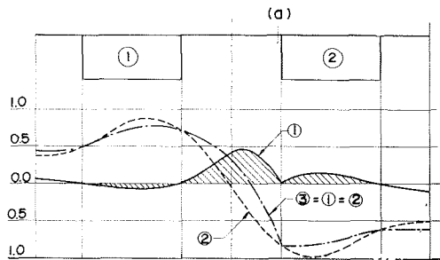
Fig. 104. — Líneas de influencia transversal, de los momentos flectores, en la losa.
