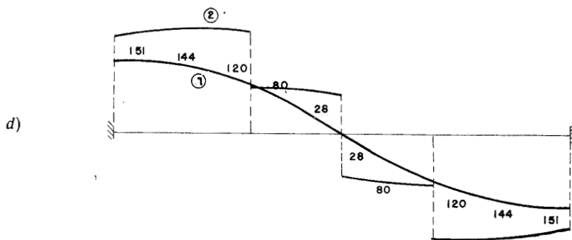
Fig. 101. — Tramo empotrado L = 80 \text{ m} .
