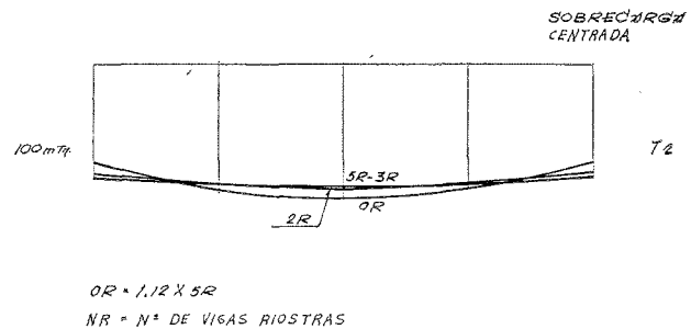
Fig. 36.—Distribución momentos flectores centro viga empotrada-centrada.
