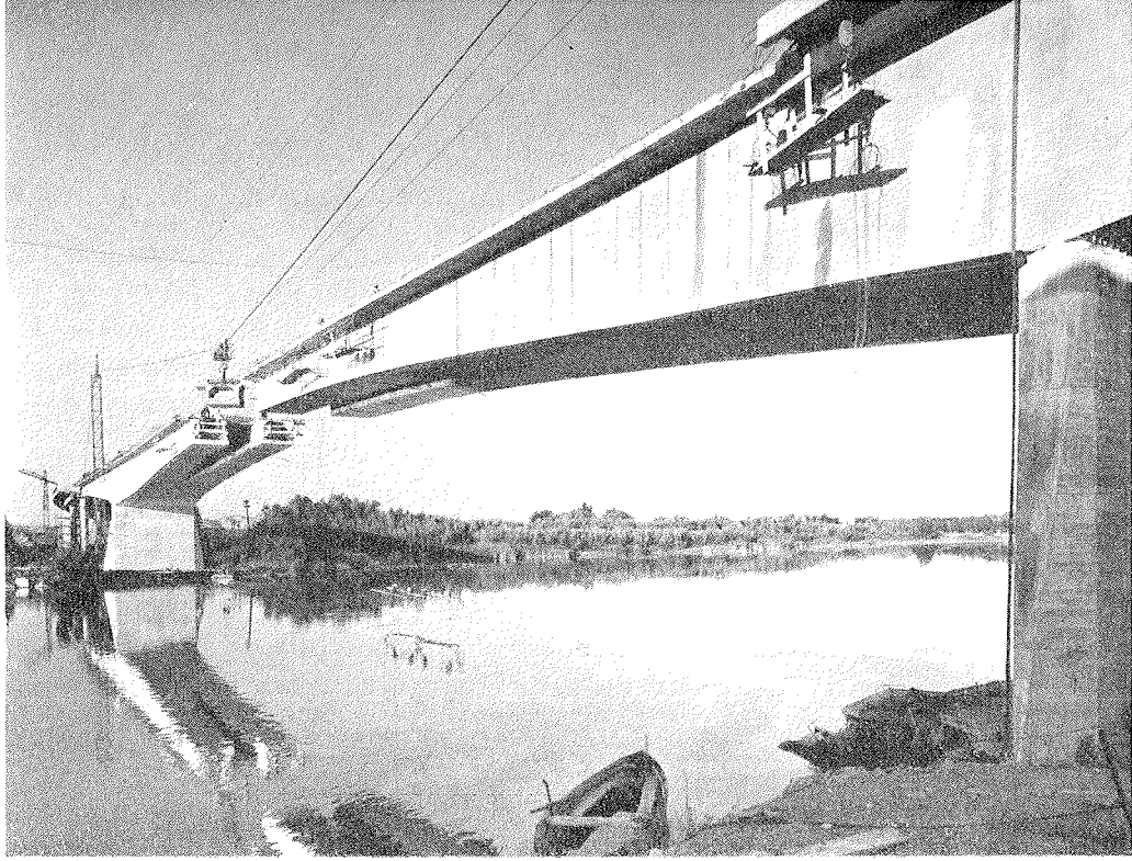
Puente de Castejón sobre el Ebro. Colocación de una dave'a prefabricada (1968).
