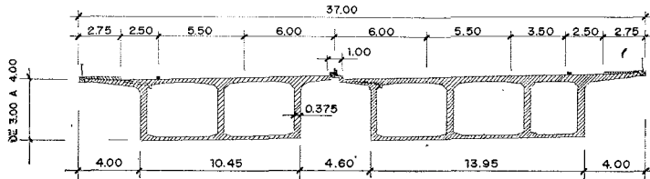
Fig. 125. — Puentes del zoo de Coloma (1965).
