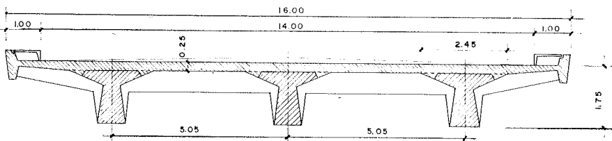
Fig. 68. — Viaducto Docciola (1965).
