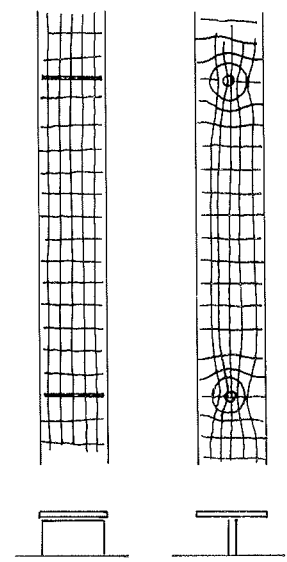
Fig. 2. — Variación de la relación: ancho/luz.
