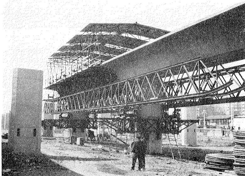
Fig. 5. — Puente de ferrocarril en Gerona. Cimbra autoportante. Ciclo completo (encofrado-armado-hormigonado-pretensado y traslado de la cimbra al vano siguiente), cuatro días (1970).
