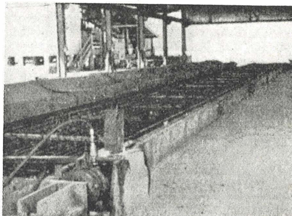
Fig. 3. Banco especial para producción de traviesas pretensadas.
