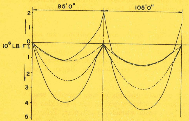
--- CARGA PERMANENTE (SOLAMENTE DE LA VIGA) - - - " " (VIGA Y LOSA "IN SITU") — ENVOLVENTE DE MOMENTOS FLECTORES (INCLUYENDO SOBRECARGA)
