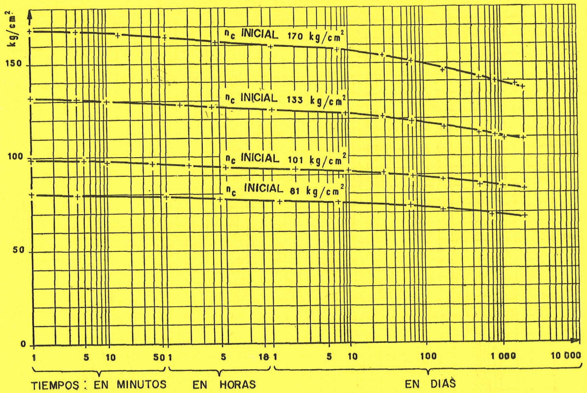
Fig. 6.—Variación de la tensión de compresión en el hormigón, en función del tiempo.—Hormigón cargado al año de edad, con alambres trejados.
