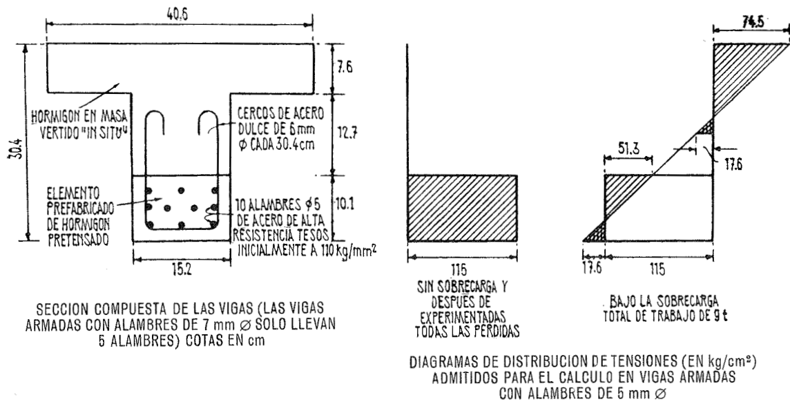
Fig. 3.—Vigas de hormigón pretensado para los ensayos de fatiga.
