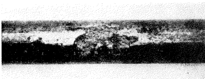
Figs. 2 y 3.—Secciones de alambres en las que puede apreciarse la rotura con lúnula
