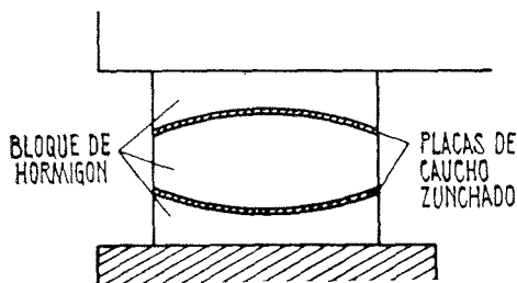
Fig. 4.—Rótula de apoyo.
