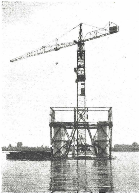
Construcción de los soportes circulares de coronación de una de las pilas. Pueden verse los elementos metálicos que servirán después para soportar la cimbra de las vigas en ménsula.
