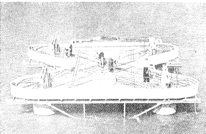
Construcción de una de las placas de hormigón armado, de 60 cm de espesor, que enlaza las cabezas de los pilotes de cimentación de las pilas.
