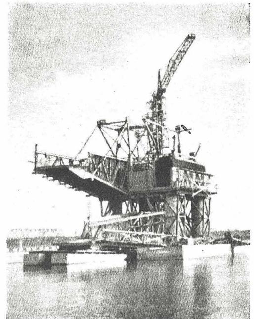
Construcción de los soportes circulares de coronación de una de las pilas. Pueden verse los elementos metálicos que servirán después para soportar la cimbra de las vigas en ménsula.
