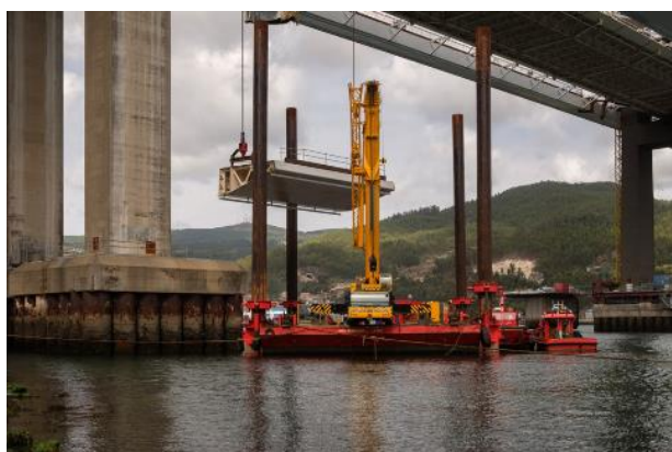
Figura 7.- Detalle de izado de dovela lateral lado Sur desde pontona
