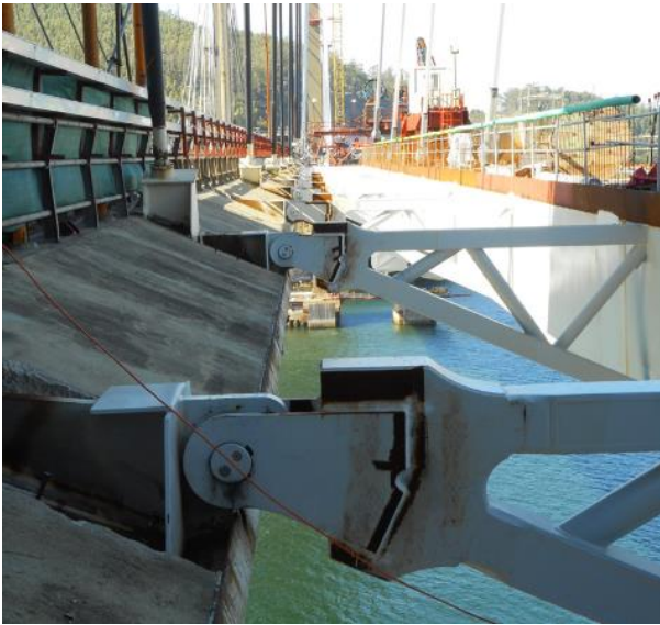
Figura 3.-Detalle de union de la rótula y la dovela
