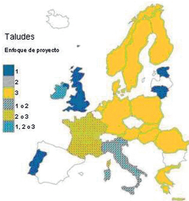
Figura 14. Enfoques de Proyecto elegidos en los Anejos Nacionales de los diferentes países europeos para la estabilidad global y de taludes (Tomada de [16]).
