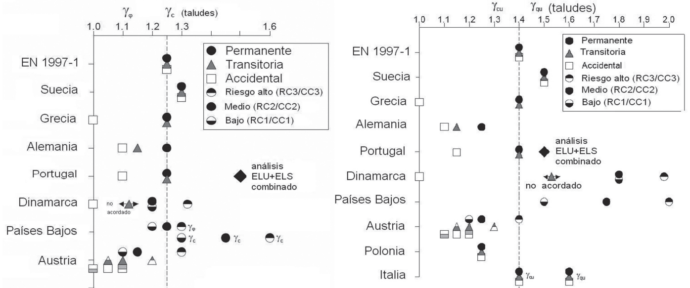
Figura 15. Coeficientes parciales de minoración del ángulo de rozamiento ( \gamma_\phi ) y la cohesión ( \gamma_c ) efectivos (fig. 10A) y de la resistencia al corte no drenada ( \gamma_{qu} ) (fig. 10B) adoptados por diferentes anejos nacionales europeos [16].
