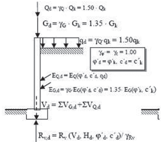
Figura 2. Método de mayoración de acciones para la verificación del estado límite de hundimiento de una cimentación superficial (por simplicidad, solo se muestran las acciones verticales desfavorables) (Tomada de [8]).
