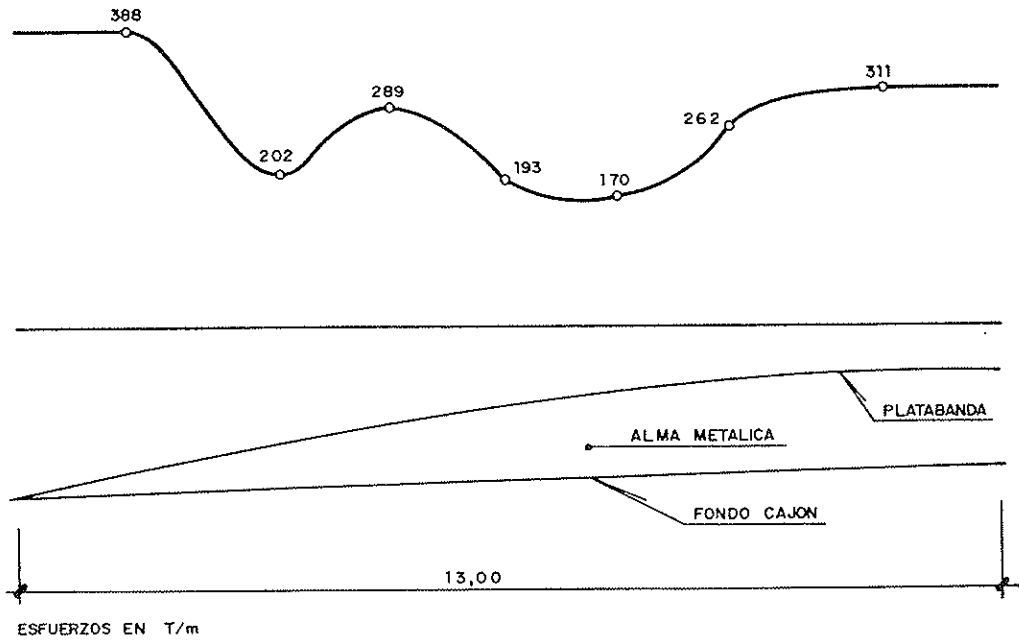
Fig. 25. Envolvente esfuerzos rasantes en zona de conexión.
