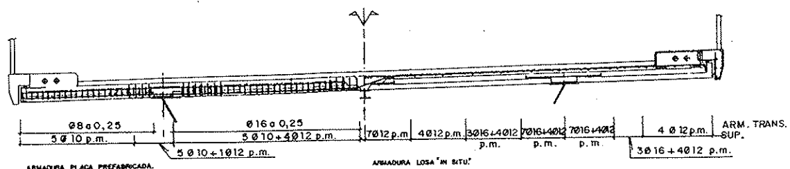
Fig. 8. Armado de la Losa y Placas Prefabricadas.
