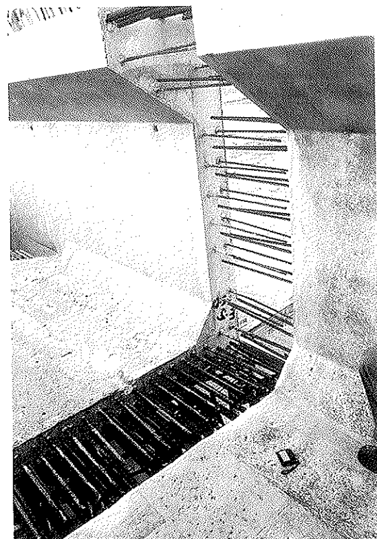
Fig. 8. Junta húmeda.
