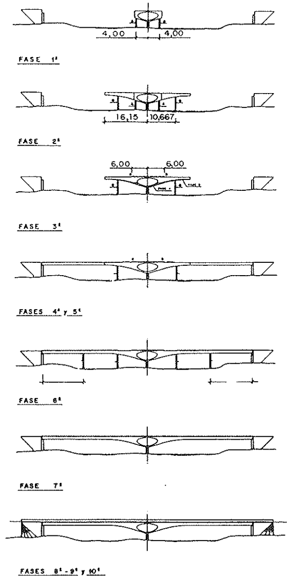
Fig. 22. Proceso de Montaje.
