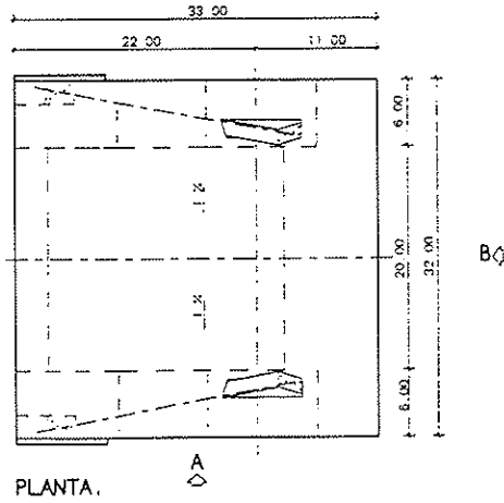
Figura 2. Contrapeso 1. Geometría.
