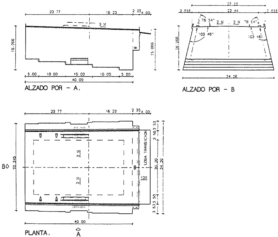
Figura 3. Contrapeso 2. Geometría.
