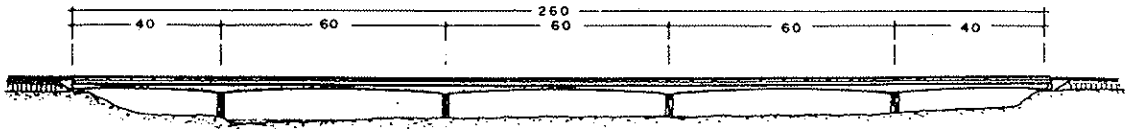
Fig. 2. Alzado General.
