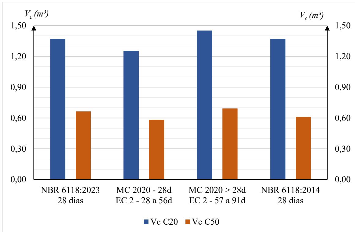
Figura 2.3. Gráfico de barras que indica el volumen de hormigón correspondiente a cada alternativa de diseño del tramo de pilar, para una cuantía mínima de armadura ( \geq 0,4\% ).
